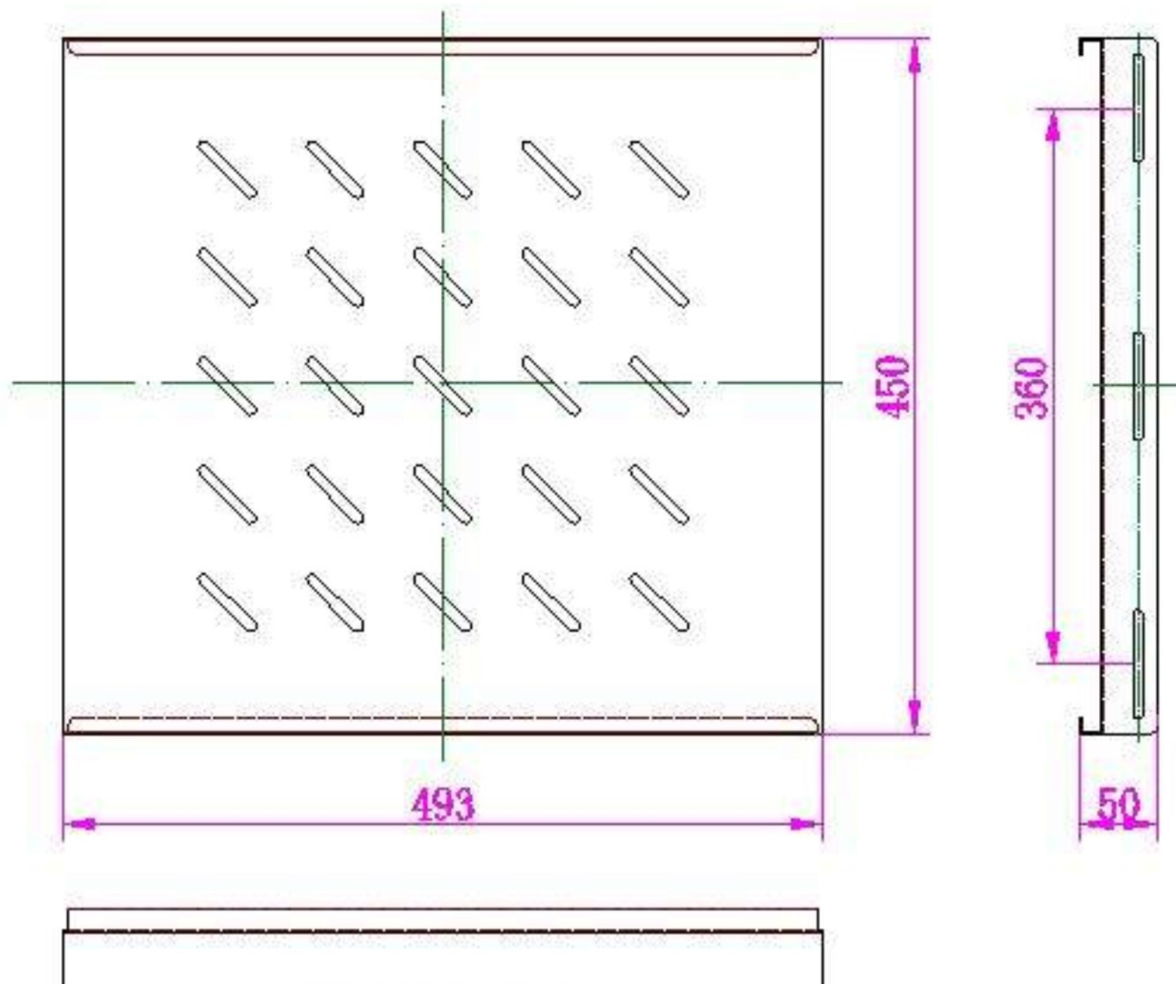
450深固定层板
